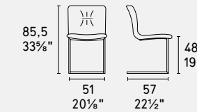
CS1849 CS1849-MTO
